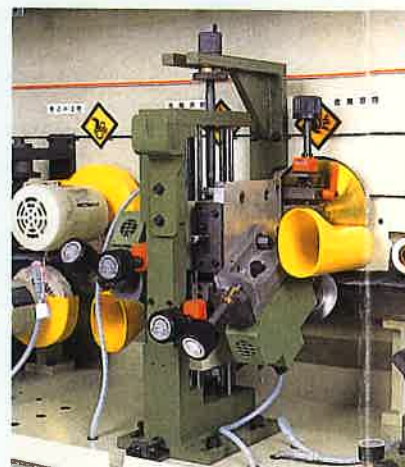
● トリミング装置
